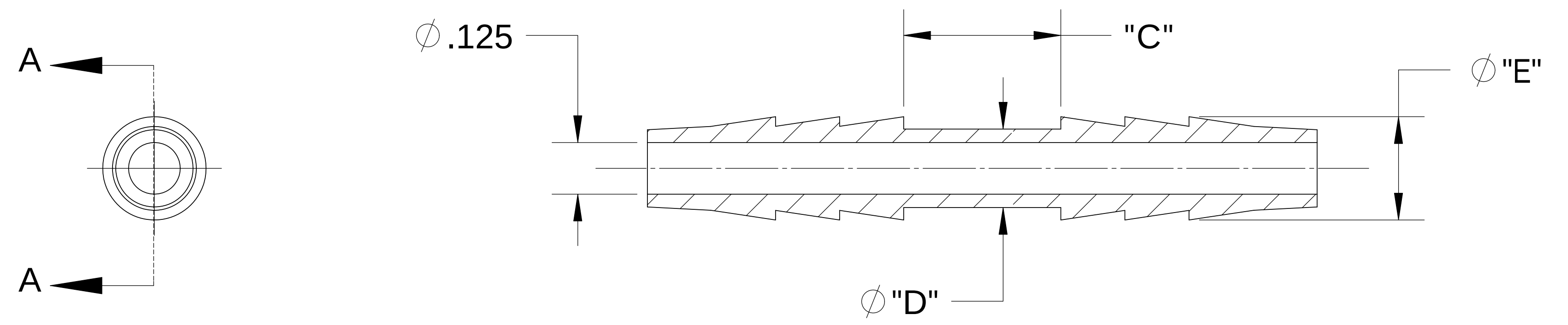
SECTION A-A
