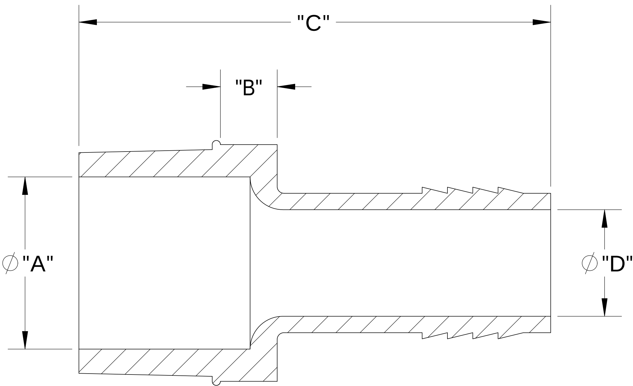
SECTION A-A
