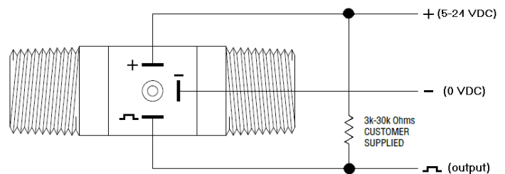
DIN Output
