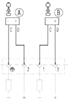
Anschluss Schaltbild
