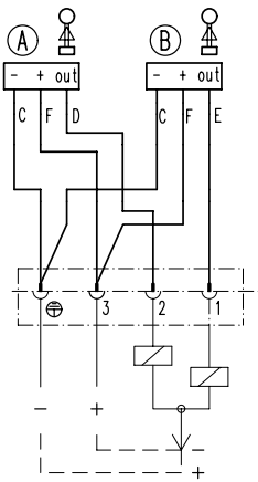
Anschluss Schaltbild
