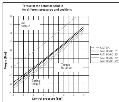
PA 21 Drehmomentkennlinie
