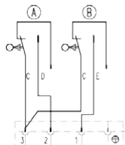
Anschluss Schaltbild
