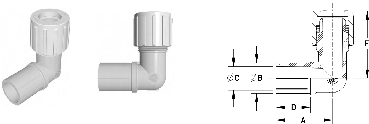
Furon® ETA Elbow Tube Adapter
