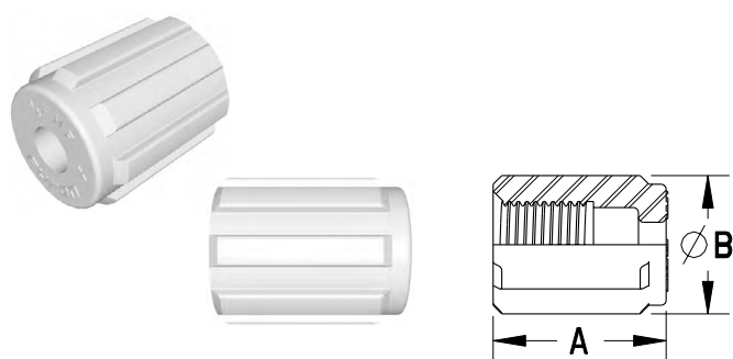
Furon® PFA Nut
