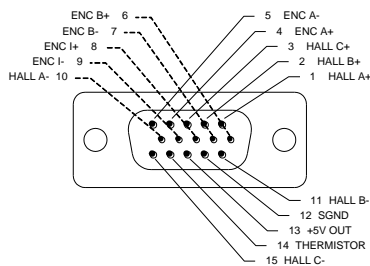
Incremental Encoder
